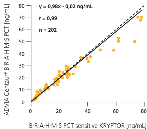
Corrélation entre B-R-A-H-M-S PCT sensitive KRYPTOR et ADVIA Centaur® B-R-A-H-M-S PCT mesuré sur l'automate ADVIA Centaur® CP
