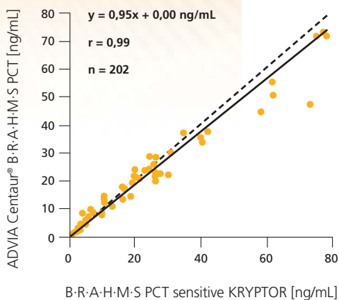
Corrélation entre B-R-A-H-M-S PCT sensitive KRYPTOR et ADVIA Centaur® B-R-A-H-M-S PCT mesuré sur l'automate ADVIA Centaur® XP
