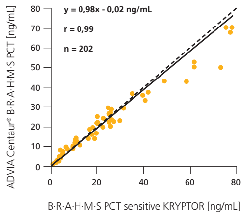
Korrelation zwischen B·R·A·H·M·S PCT sensitive KRYPTOR und ADVIA Centaur® B·R·A·H·M·S PCT gemessen auf dem ADVIA Centaur® CP Analyzer
