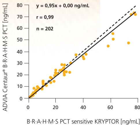
Korrelation zwischen B·R·A·H·M·S PCT sensitive KRYPTOR und ADVIA Centaur® B·R·A·H·M·S PCT gemessen auf dem ADVIA Centaur® XP Analyzer
